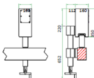
Инспекционная голова с камерой
